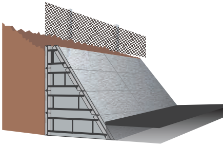
山留に 落石防護柵設置
