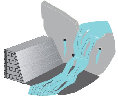
砂防堰堤の放流路に
