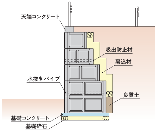
■ 重力式 直積み擁壁タイプ
