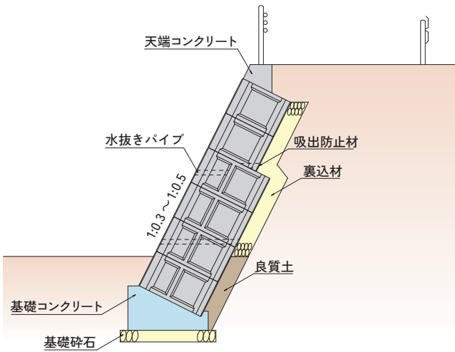
■ もたれ式 重ね積み擁壁タイプ
