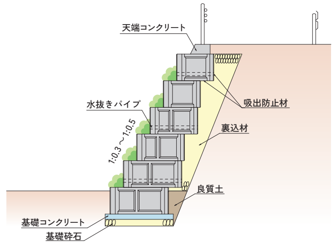
■ もたれ式 階段積み擁壁タイプ
