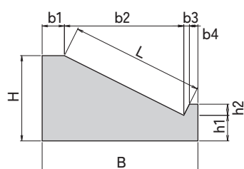
(もたれ式重ね積み擁壁タイプ)
