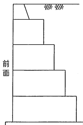
重力式重ね積み擁壁
