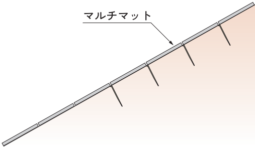
■ 標準施工断面図
