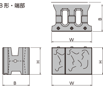
■ B形・端部
