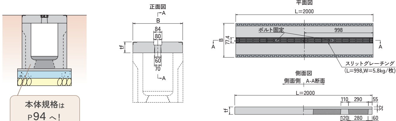
■ 規格寸法表
