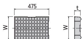
平面図
