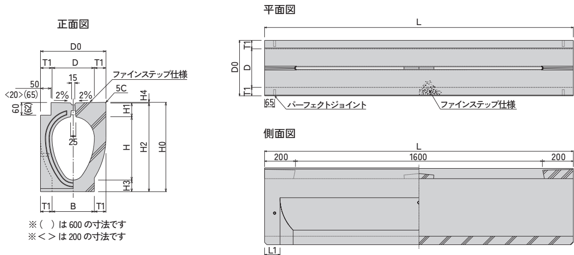
■ 規格寸法表
