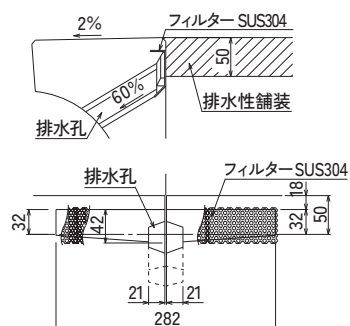
排水孔詳細図
