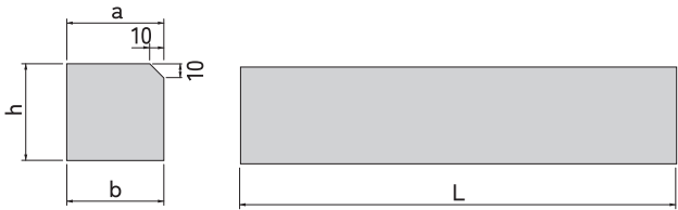
■ 規格寸法表
