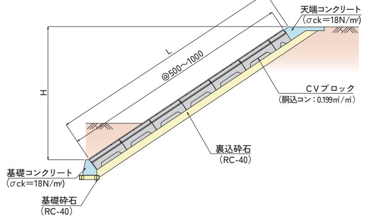
■ 緩傾斜施工断面図
