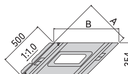
側面図
