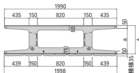
C-C 矢視図
