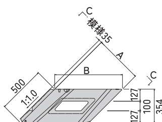
A-A 断面図
