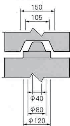
B-B詳細図
