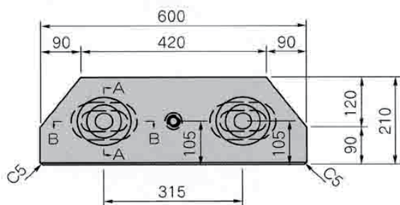
平面図
