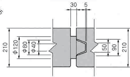
A-A詳細図
