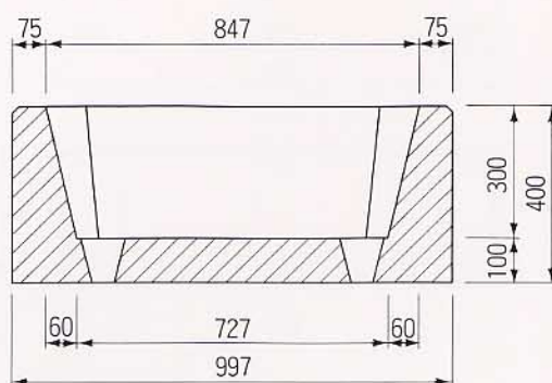
A-A断面図
