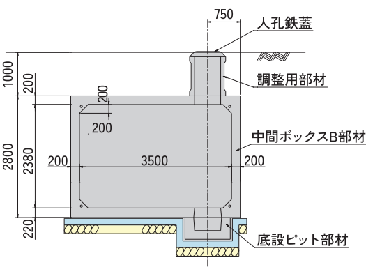
■ A-A断面図
