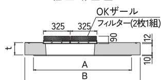
組立断面図
