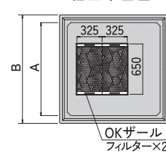
組立平面図
