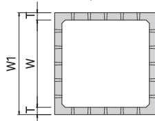
平面図
