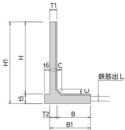
■ L 型水路 規格寸法図
