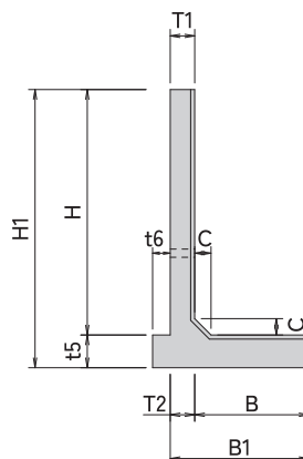
■ 逆 L 型擁壁 規格寸法図
