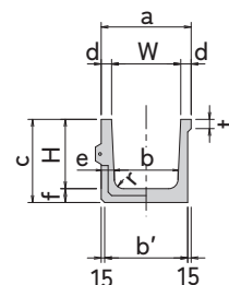
正面図（下流側）
