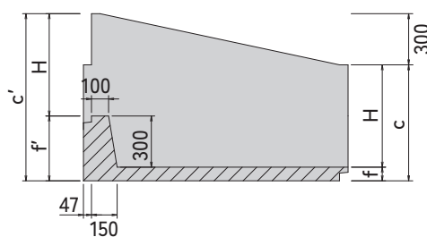
断面図
