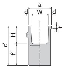
正面図（上流側）
