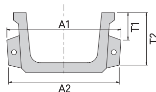
ボルト連結部寸法
